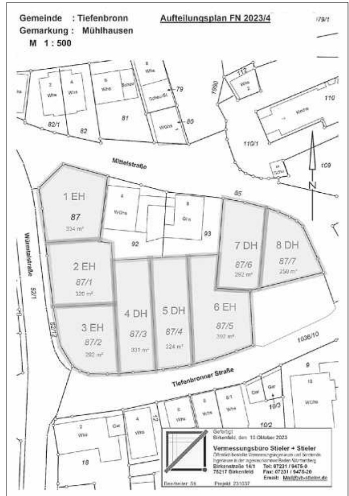
Zeichnerischer Plan
